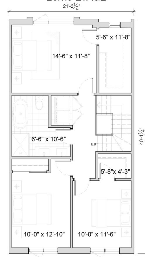
2ème ÉTAGE
