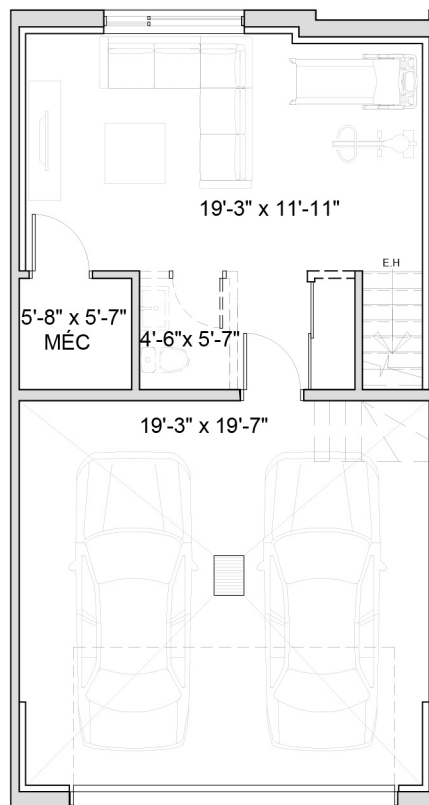
SOUS-SOL
